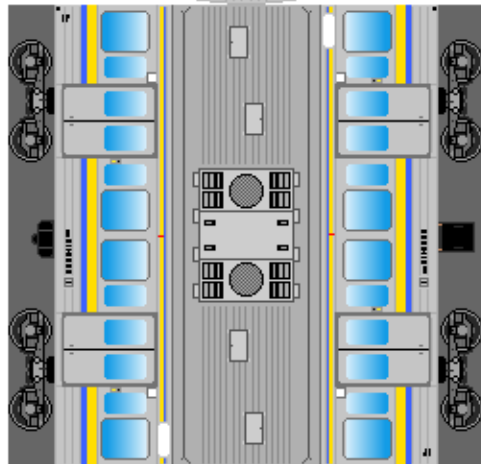
④ サハ211
