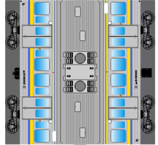
③ サハ211
