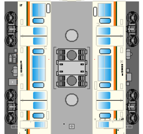
⑩ クハ103
