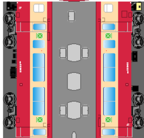
⑦ サロ455
