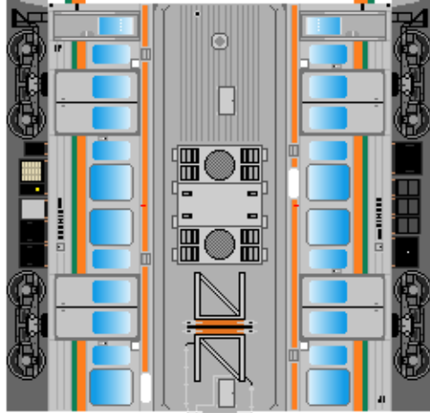
① クモハ211
