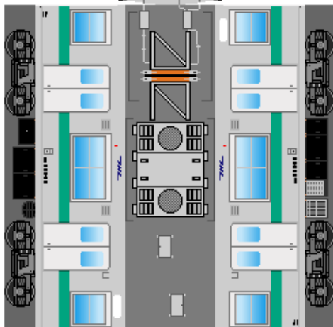
③ モハ203
