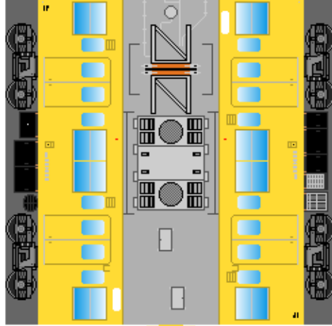
② モハ201
