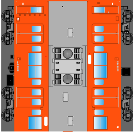
⑦ クハ201
