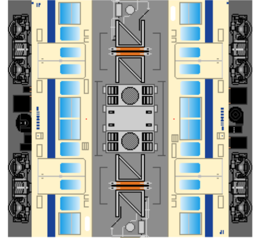
③ モハ114
