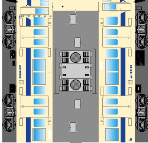
① クハ115
