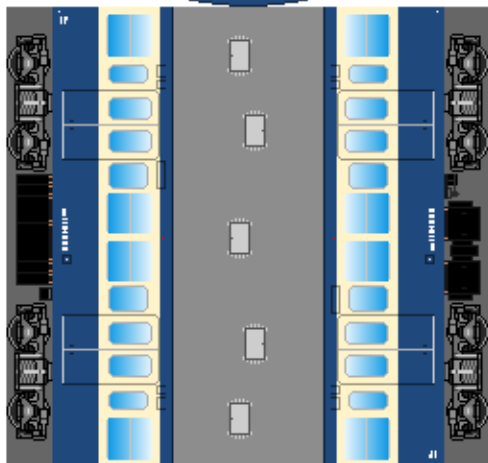
③ モハ113
