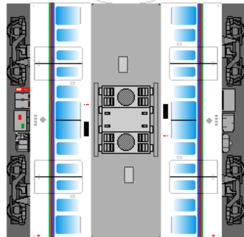
3号車 モハ (偶数)
