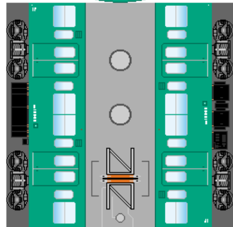
② モハ103
